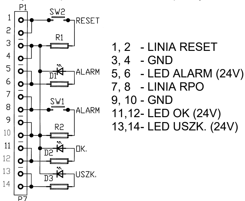
Rys.2. Schemat elektryczny przycisku RPO1.
