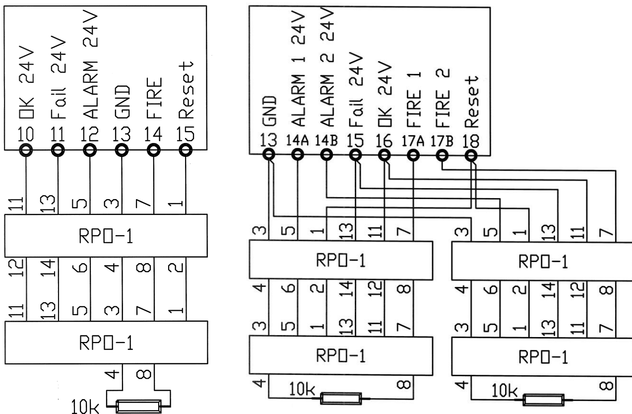
Rys.3. Schemat połączeń przycisku mcr RPO-1a z centralą SVM (z lewej) oraz SV (z prawej).
